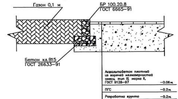
Конструкция тротуарного покрытия для новых дорожек
