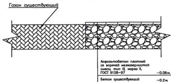
Конструкция тротуарного покрытия существующего
